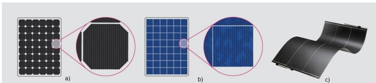
a) Painel Solar Monocristalino, b) Painel Solar Policristalino, c) Painel Solar de Filme Fino
